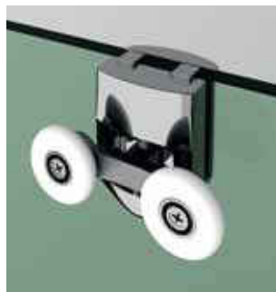
Rodamiento superior con tornillo de regulacion
