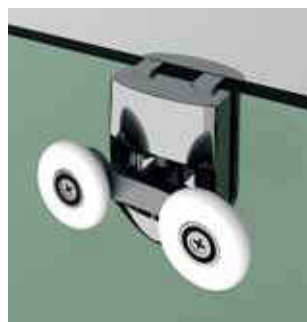
Rodamiento superior con tornillo de regulación
